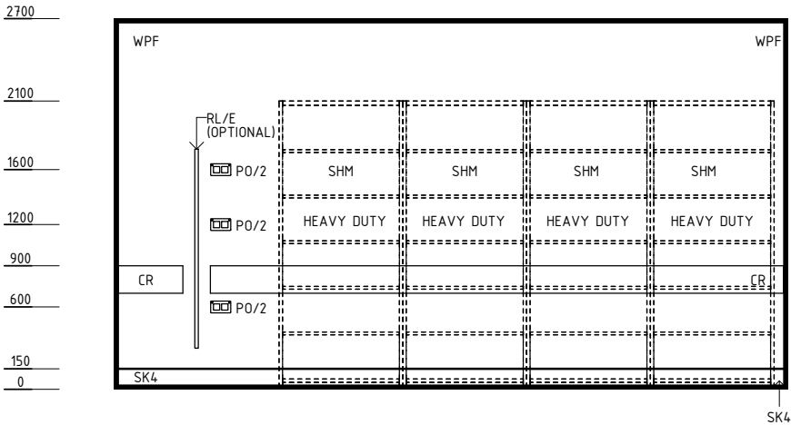
ELEVATION 4
