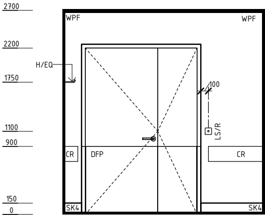
ELEVATION 3
