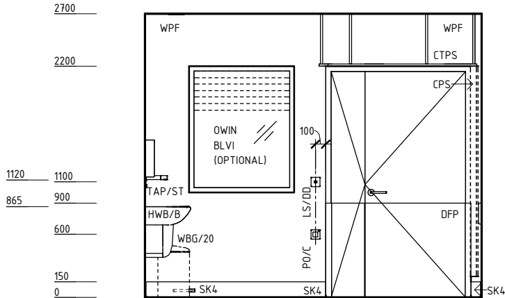
ELEVATION 3
