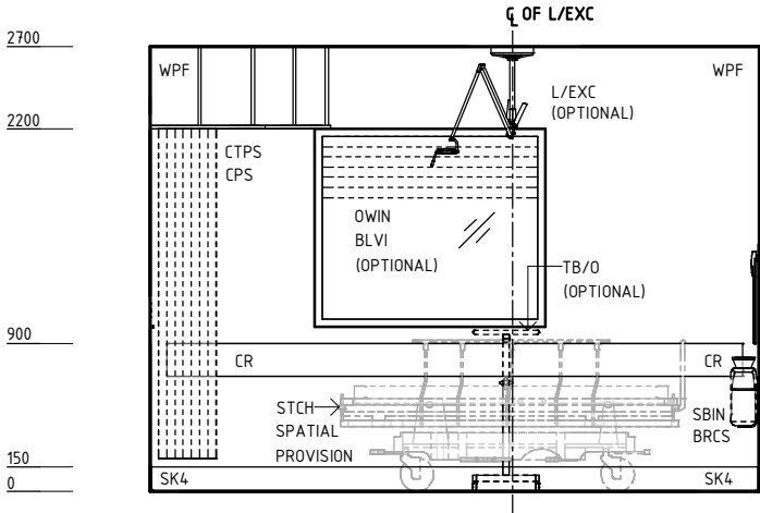
ELEVATION 4
