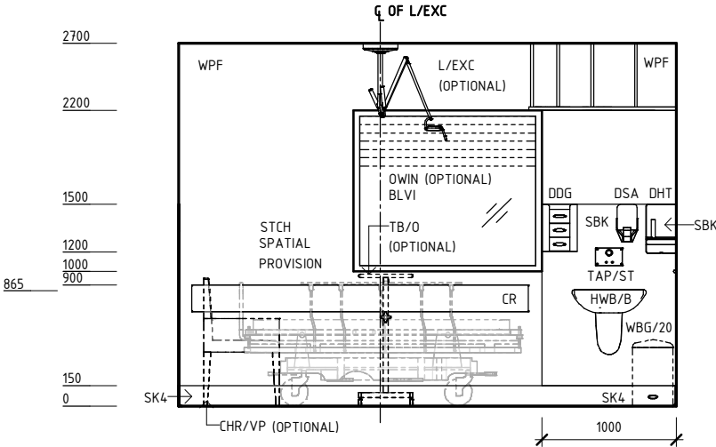
ELEVATION 2
