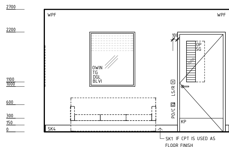
ELEVATION 3
