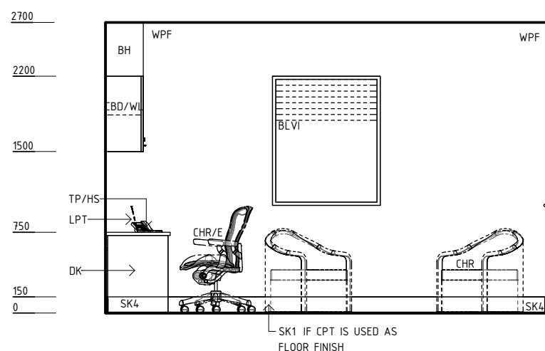
ELEVATION 1
