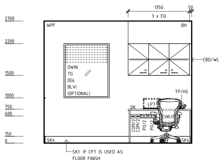
ELEVATION 4
