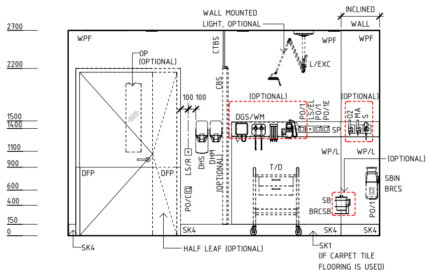
ELEVATION 3
