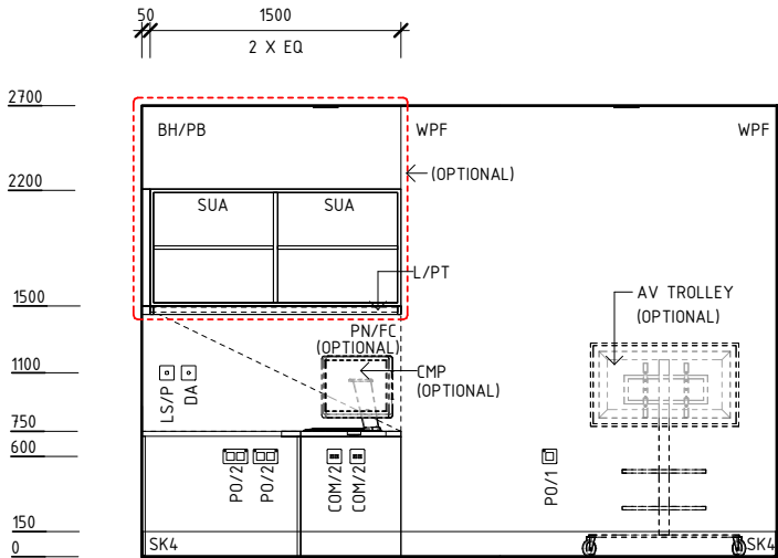
ELEVATION 2
