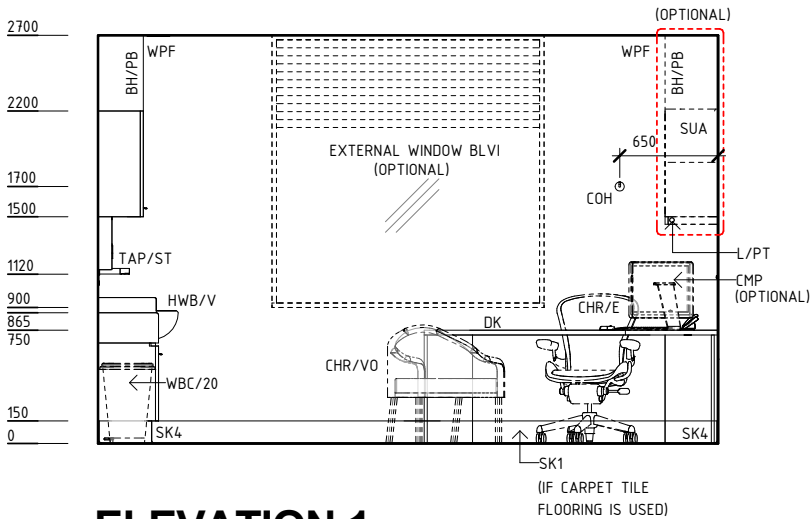
ELEVATION 1
