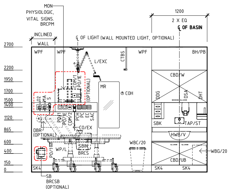
ELEVATION 4
