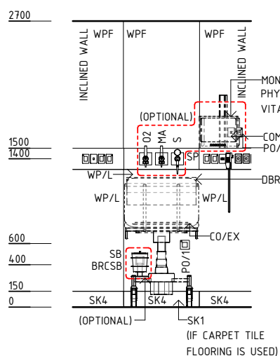
ELEVATION 5
